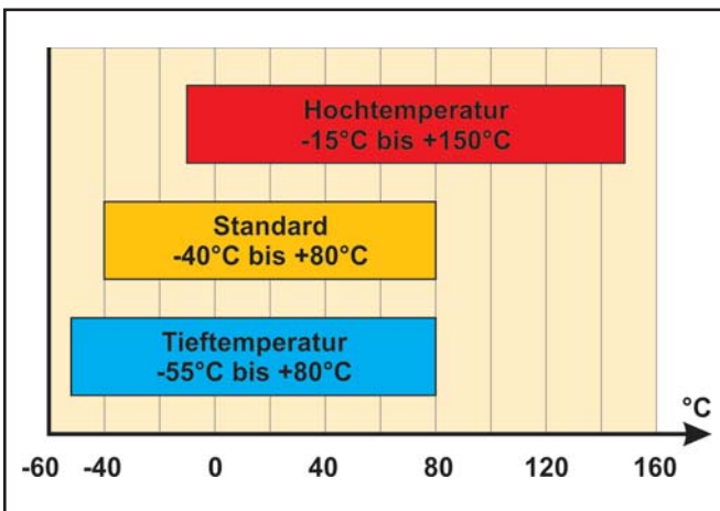
Bild 4 - Temperaturbereich
