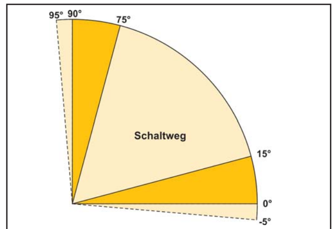
Bild 6 - Einstellbereich
