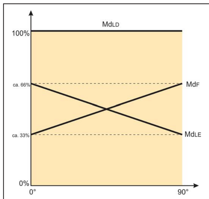
Bild 3 - Drehmomentverlauf bei empfohlenem Zuluftdruck
