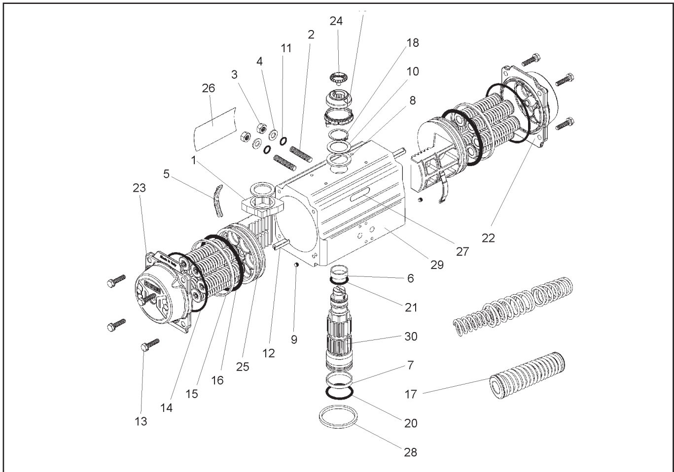
Bild 9 - Explosionszeichnung des Schwenkantriebs BR 31a
