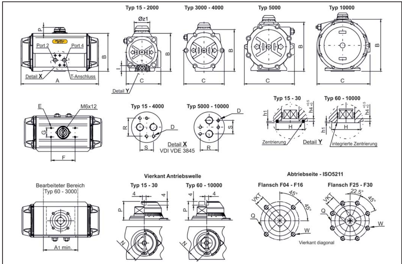
Bild 8 - Maßzeichnung des Schwenkantriebs BR 31a
